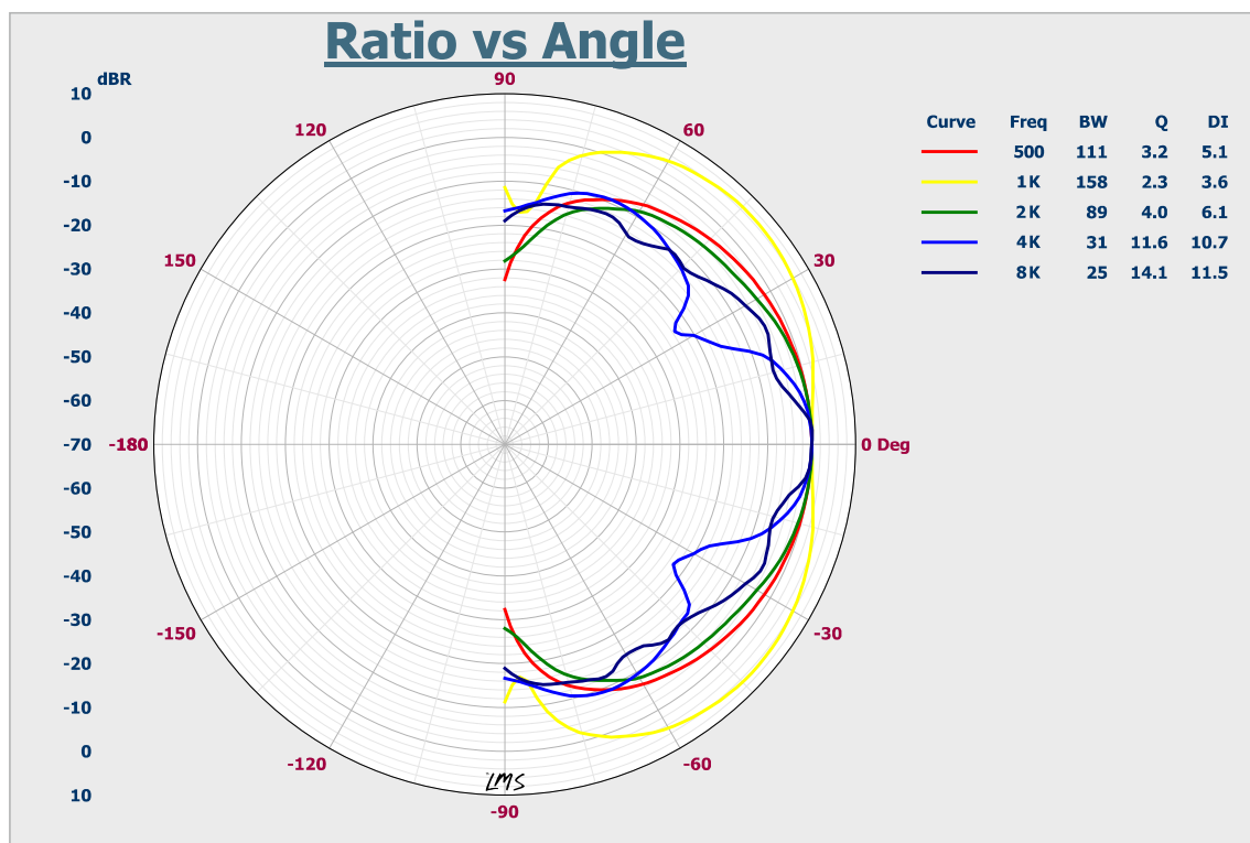
Круговая диаграмма направленности громкоговорителя LPA-06CL22
